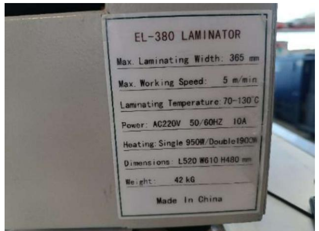
Laminadora VANSDA Thermal EL-380
