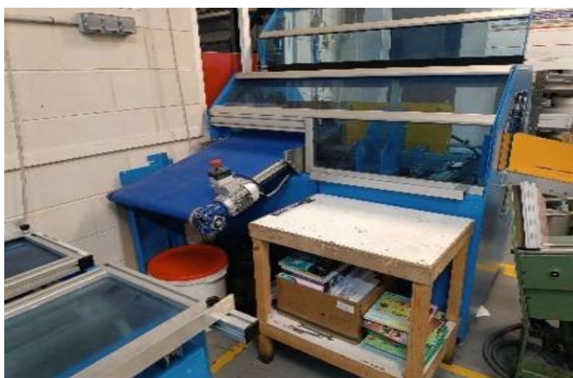
Línea de confección libros de tapa dura ZECHINI modelo X-BOOK CASE
